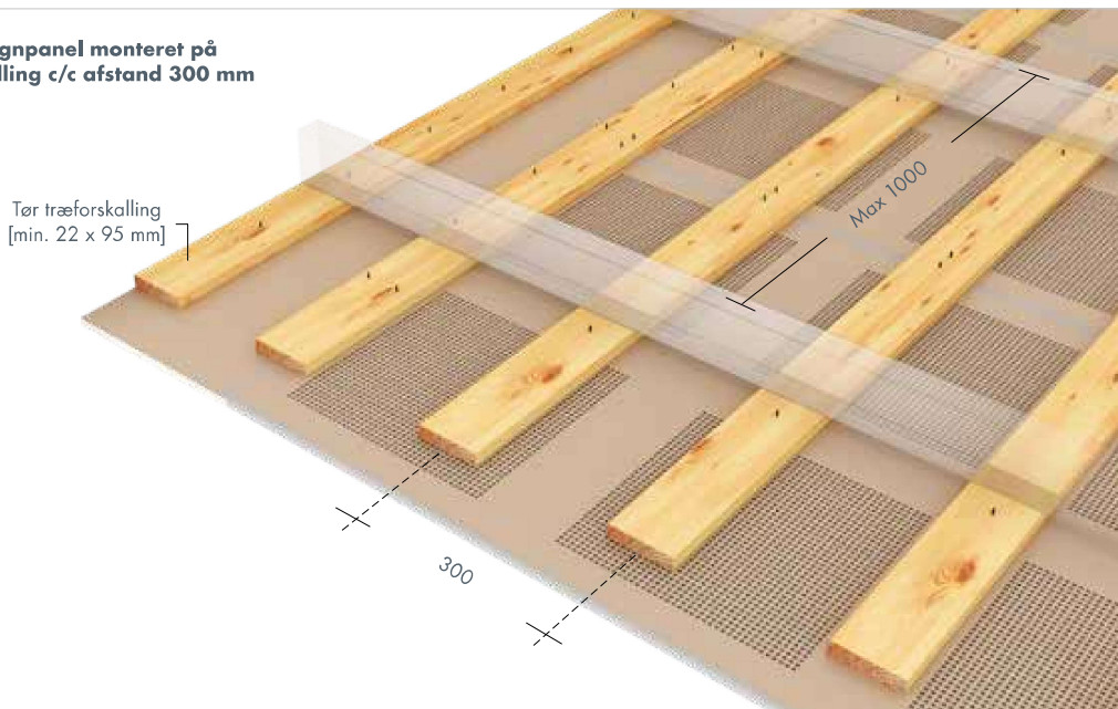
Underlagsafstande og egenvægt for pladebredde 900 og 1200 mm
