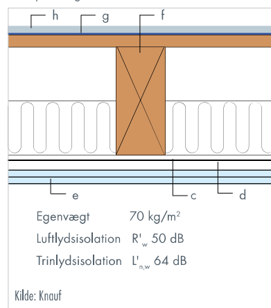
Træbjælkelag
