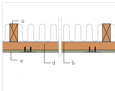
Designpanel med 50 mm forskalling
