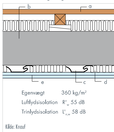
Betondæk med strøgulv og underloft
