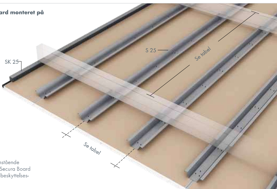
Underlagsafstande og egenvægt for pladebredde 900 mm
