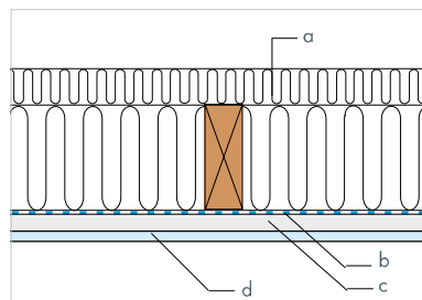
EI 30 med Secura Board
