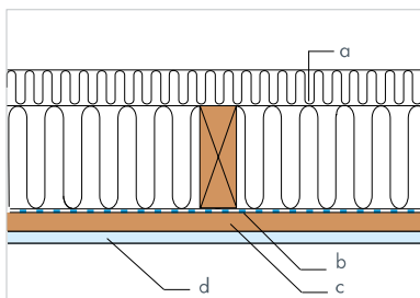
EI 30 med Classic 1 Board
